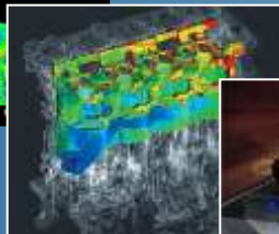
AVL-FIRE
